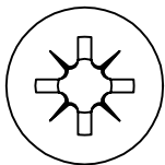
TYPE 1A (POZIDRIV®)
