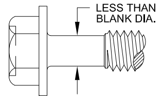
Groove
