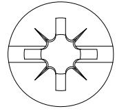
Combo Pozidriv®/Slot
